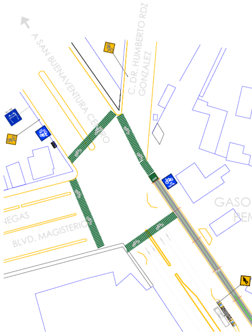
1 ENTRONQUE SAN BUENAVENTURA
