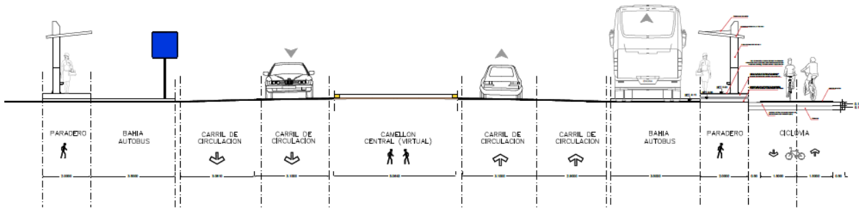
1 SECCIÓN VIALIDAD - CICLOVIA BAHIA TIPO 1 SIN ESC
