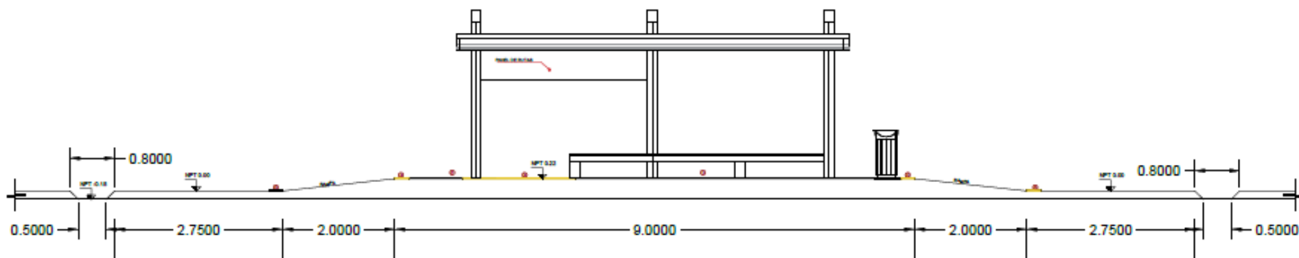
2 ELEVACIÓN ARQUITECTONICA TIPO 1 SIN ESC
